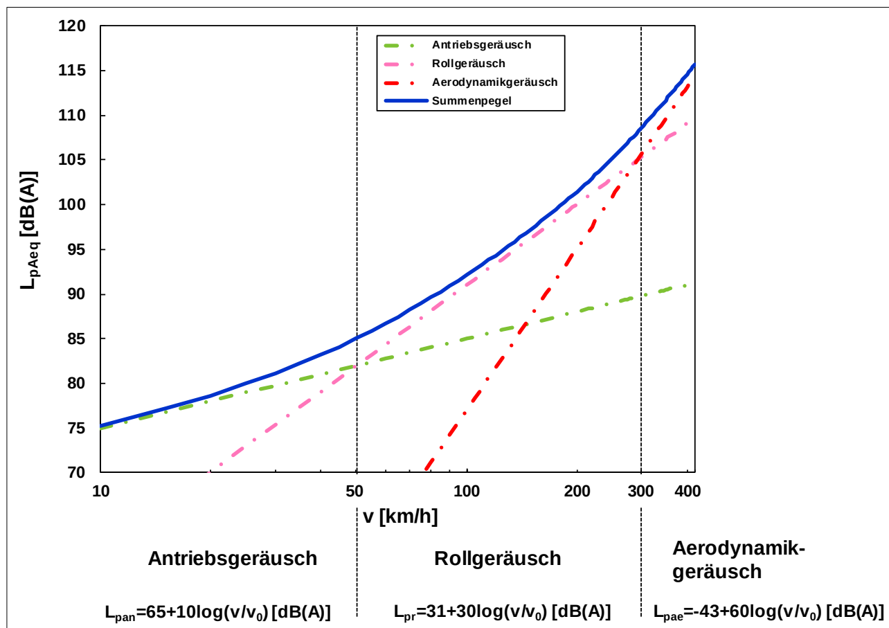
Abb. 18: Beispiel für das Geschwindigkeits-Lärmverhalten eines Triebfahrzeugs
