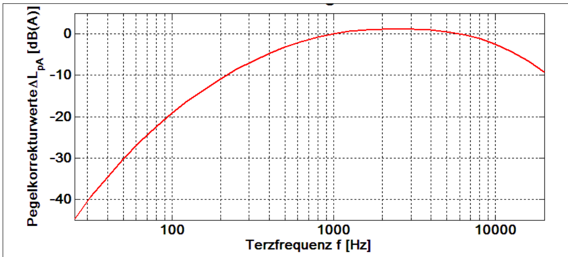
Abb. 10: A-Bewertungskurve
